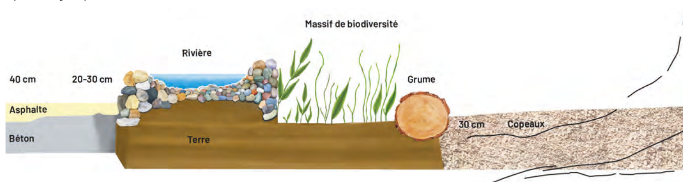
Schéma de coupe de l'aménagement de la rivière pédagogique, © a'urba
