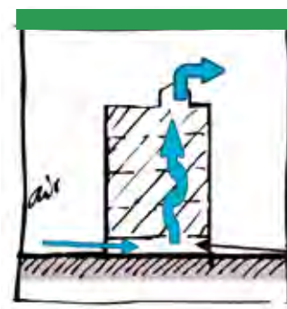
Principe de ventilation par vide sanitaire et cheminée d'aération
