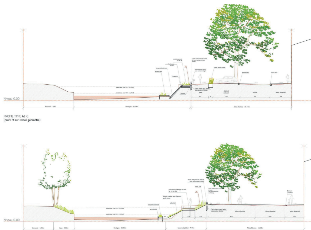
Profils du réaménagement des berges, © D'une ville à l'autre
